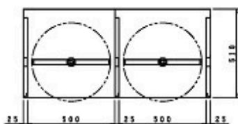
防火衣収納庫本体横断面
