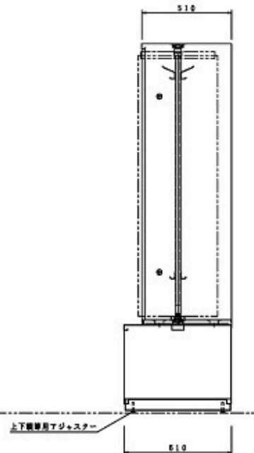
下段収納庫本体横断面
