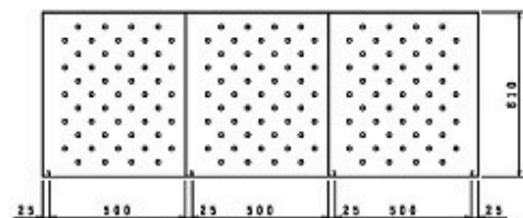
下段収納庫本体横断面
