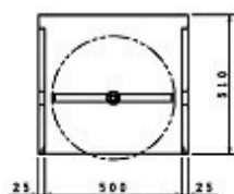
防火衣収納庫本体横断面
