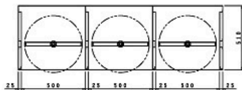
防火衣収納庫本体横断面
